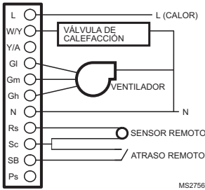
Fig. 7. Diagrama de cableado de dos tubos, solo calefacción (120/240/277 VCA en la ilustración).
