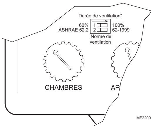
Réglage de la durée de la ventilation et de la norme de ventilation.
