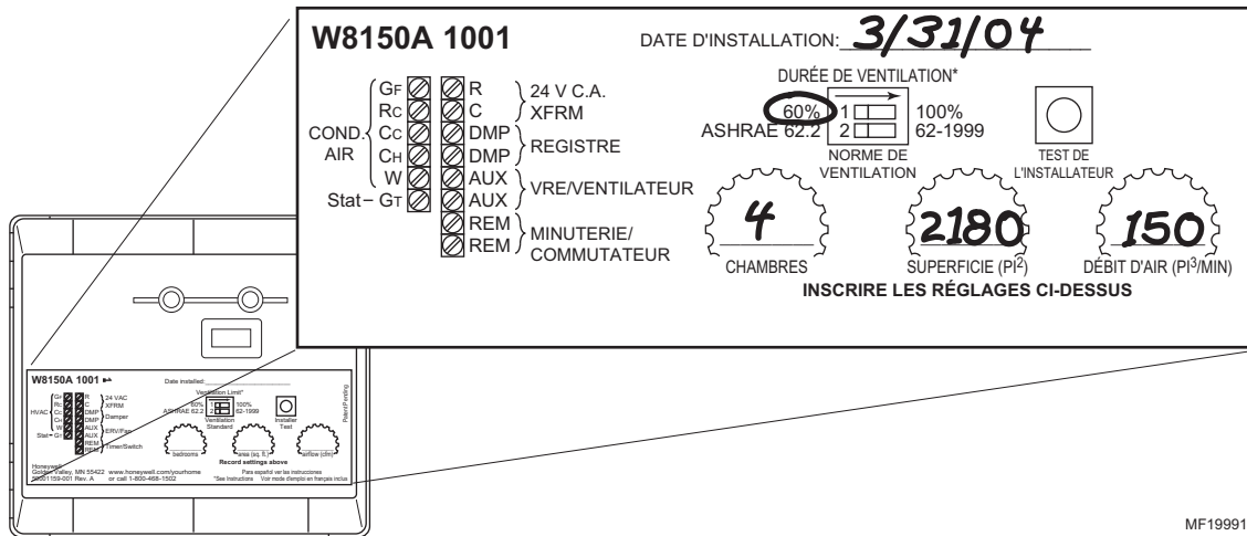
Configuration sur mesure du régulateur de ventilation.
