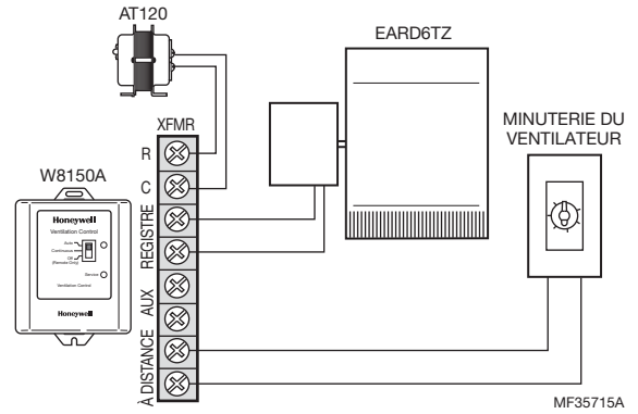
Fig. 7. Utilisation d'une commande à distance ou d'une minuterie.
