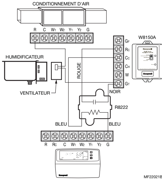
Fig. 10. Câblage d'un ventilateur pour un humidificateur à vapeur.
