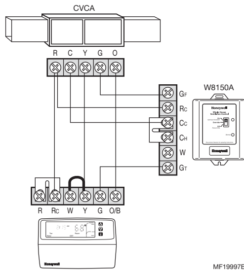
Fig. 4. Câblage d'une thermopompe sans chauffage d'urgence.
