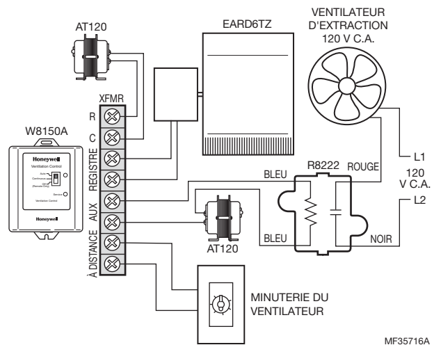
Fig. 9. Câblage d'un ventilateur d'extraction.
