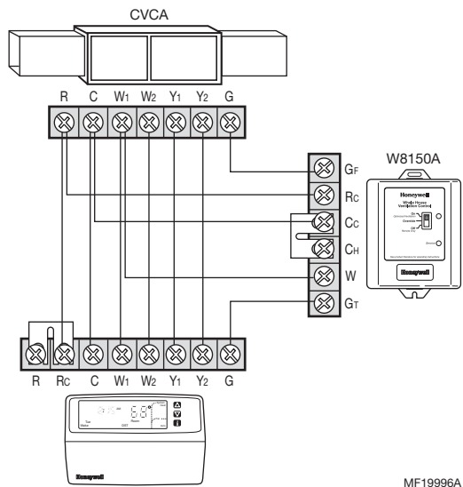
Fig. 3. Système ordinaire multi-étages.
