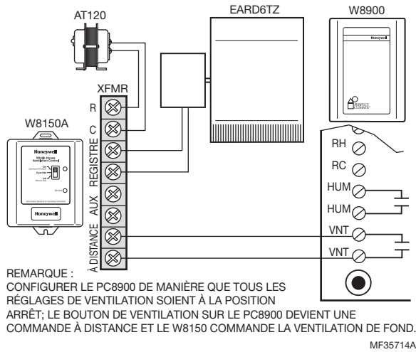
Fig. 6. Câblage avec un PC8900.
