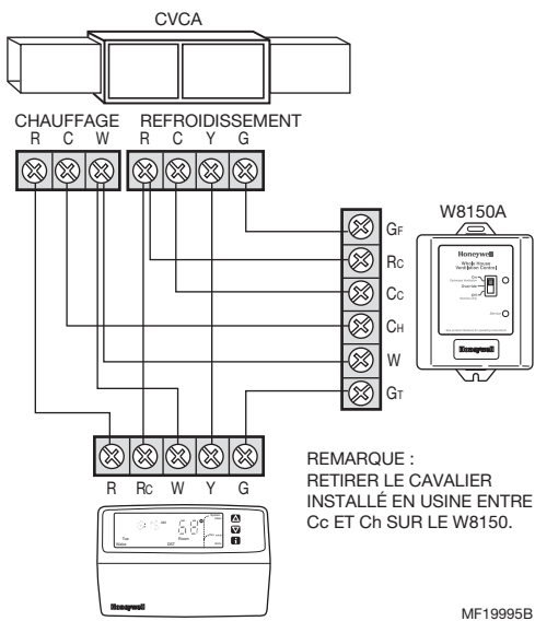
Fig. 2. Système ordinaire, deux transformateurs.
