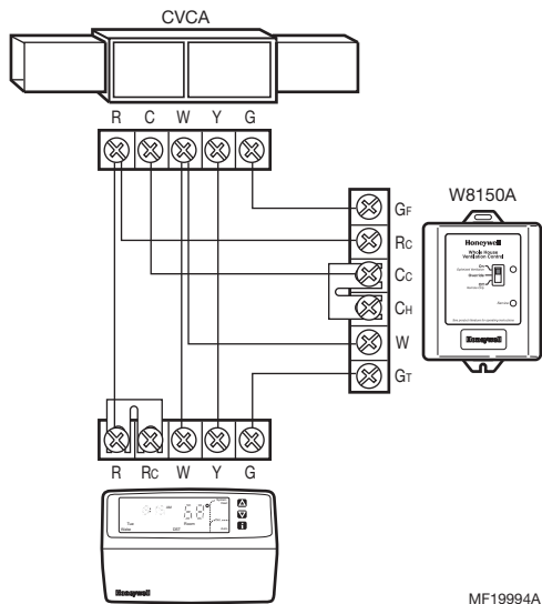
Fig. 1. Système ordinaire, un transformateur.
