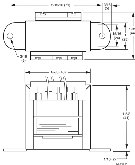
Encombrement du transformateur AT120 en mm (po).
