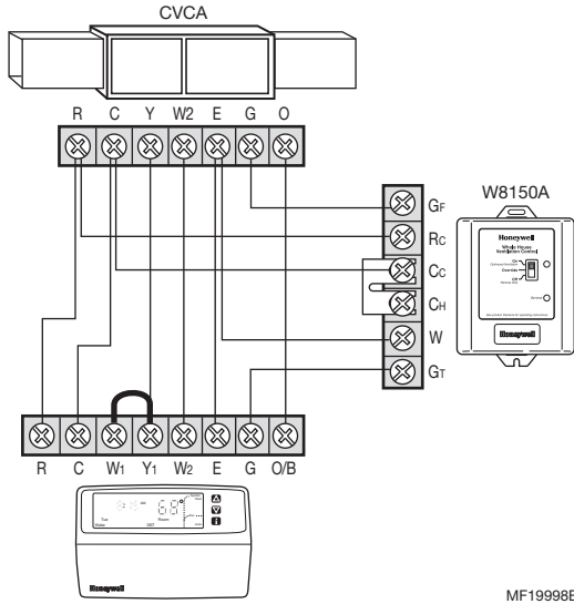
Fig. 5. Câblage d'une thermopompe avec chauffage d'urgence.
