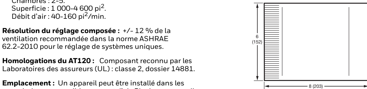
Registre EARD6TZ. Mesures en po (mm).
