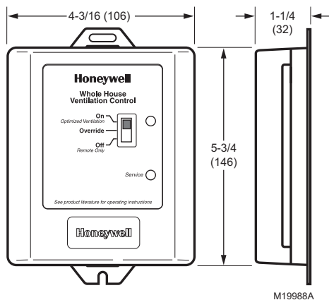
Encombrement du régulateur de ventilation W8150A en mm (po).
