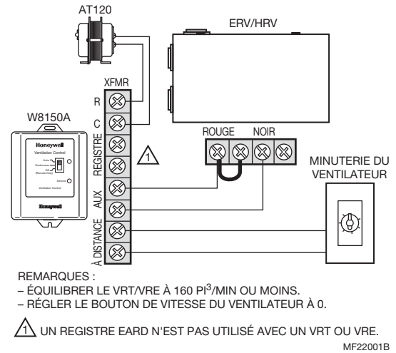
Fig. 8. Câblage à un VRT/VRE.
