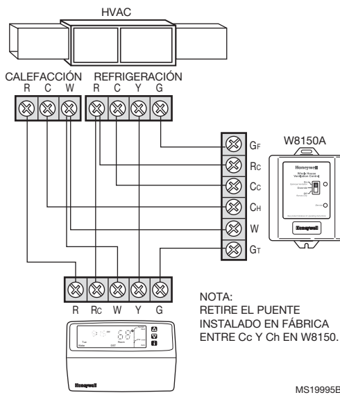
Fig. 2. Transformador doble, sistema convencional.
