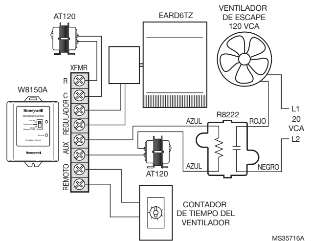
Fig. 9. Cableado de un ventilador de escape.
