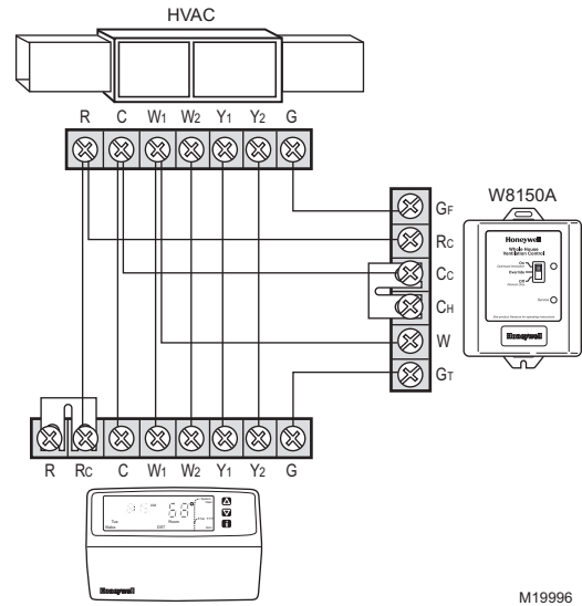
Fig. 3. Etapas múltiples, sistema convencional.
