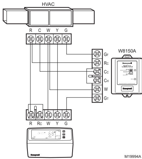
Fig. 1. Transformador individual, sistema convencional.
