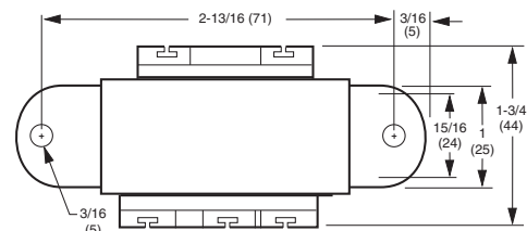
Regulador (EARD6TZ). Dimensiones en pulgadas (mm).
