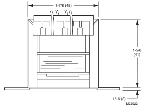
Dimensiones del transformador AT120 en pulgadas (mm).
