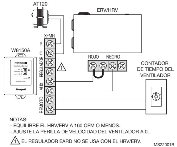
Fig. 8. Cableado a un HRV/ERV.
