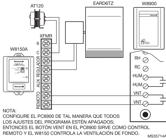
Fig. 6. Cableado con un PC8900.
