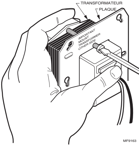
Fig. 8. Fixer la plaque sur le transformateur à l'aide de la vis de montage.
