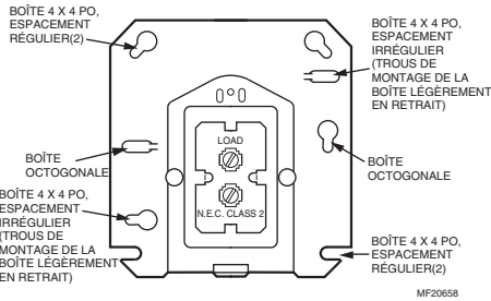
Fig. 9. Positions des trous de montage.
