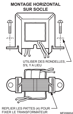
Fig. 2. Montage sur socle (modèle AT20C illustré).
