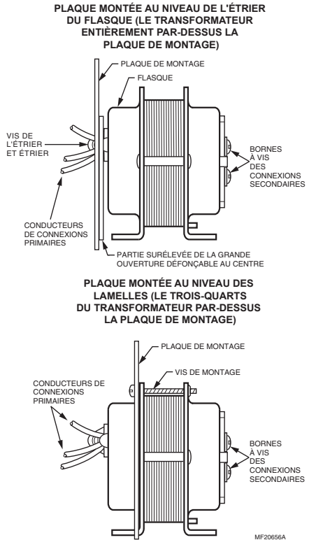
Fig. 4. La plaque peut être montée sur le transformateur dans l'une ou l'autre des positions (AT72D illustré).
