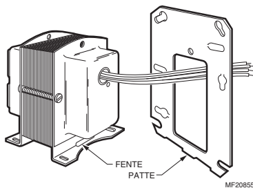
Fig. 7. Patte au centre de la plaque se glisse dans la fente du pied de montage du transformateur.
