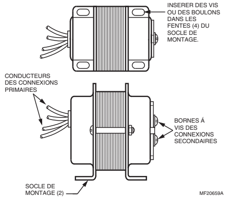
Fig. 10. Montage sur socle du transformateur AT87.
