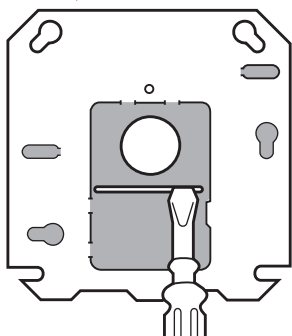
Fig. 6. Pour enlever la grande ouverture défonçable au centre.
