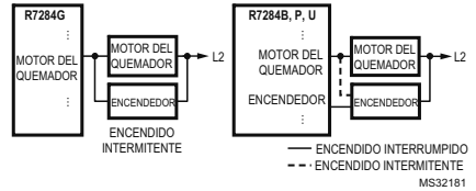
Fig. 6. Cableado del encendedor del R7284B.
