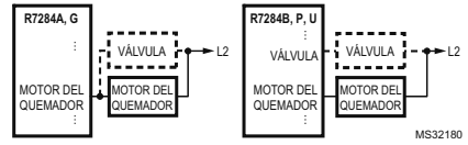
Fig. 5. Cableado para la válvula de aceite opcional del R7284B.
