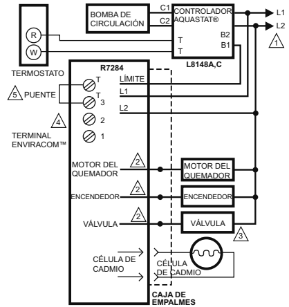
Fig. 6. Cableado del encendedor del R7284B.
